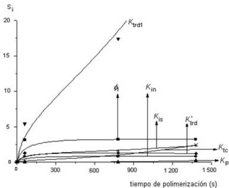
Fig. 4 Cinética de la sensibilidad ( S_i ) de los pasos elementales no despreciables en la polimerización del MF. ( \phi : rendimiento cuántico de reiniciación; k_i : iniciación radicalica; k'_{trd} : transferencia degradativa primaria; k_{is} : re-iniciación radicalica; k_p : propagación; k_{tc} : terminación cruzada alílico-acrílico).
